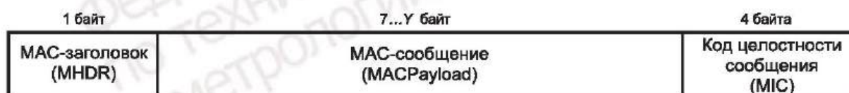
Рисунок 7 — Формат данных канального уровня восходящего сообщения
