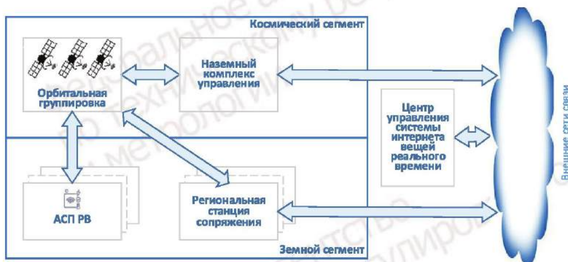
Рисунок 1 — Глобально-распределенная НСС
