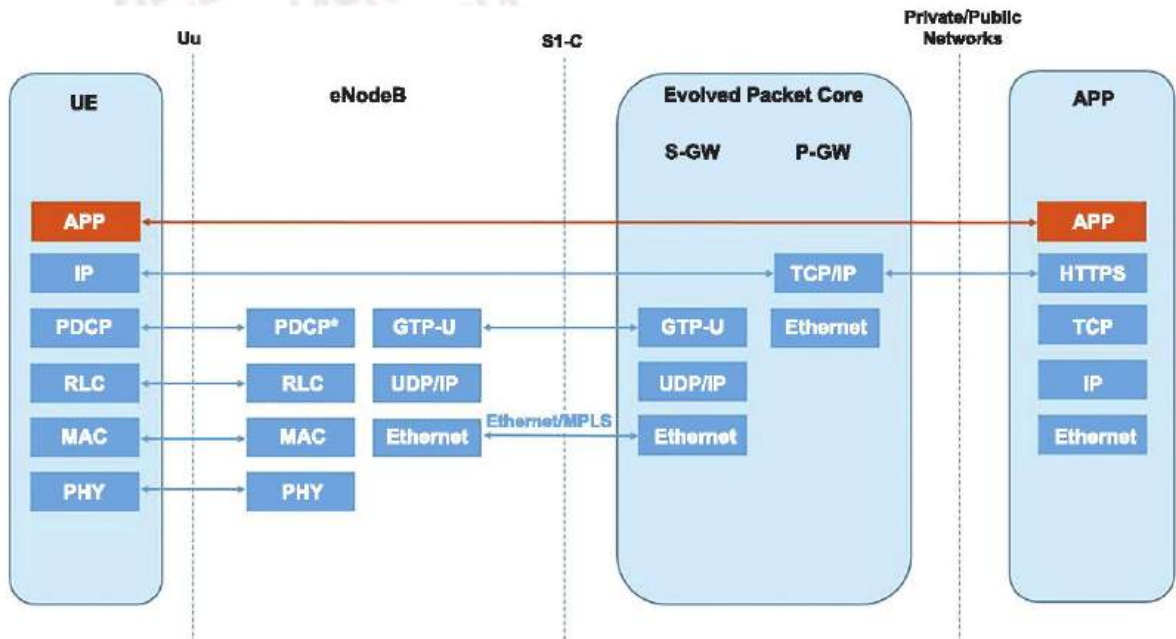
Рисунок 9 — Стек протокола передачи данных NB-IoT с использованием UP
