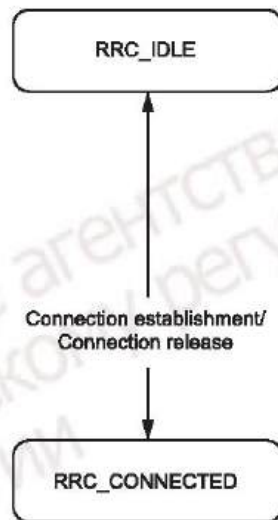
Рисунок 27 — Модель состояний уровня RRC
