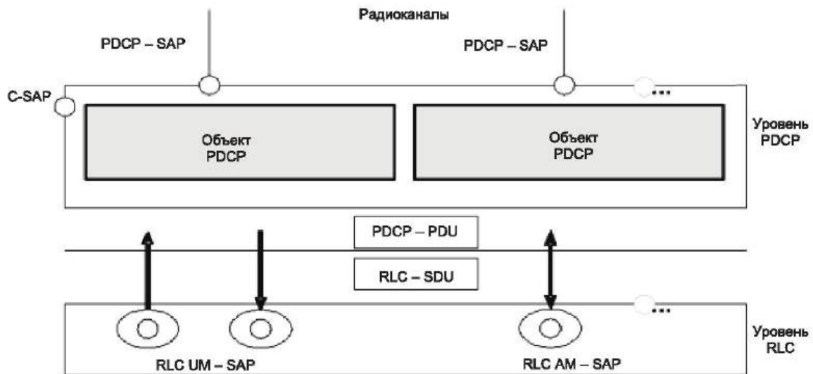
Рисунок 24 — Структура уровня PDCP
