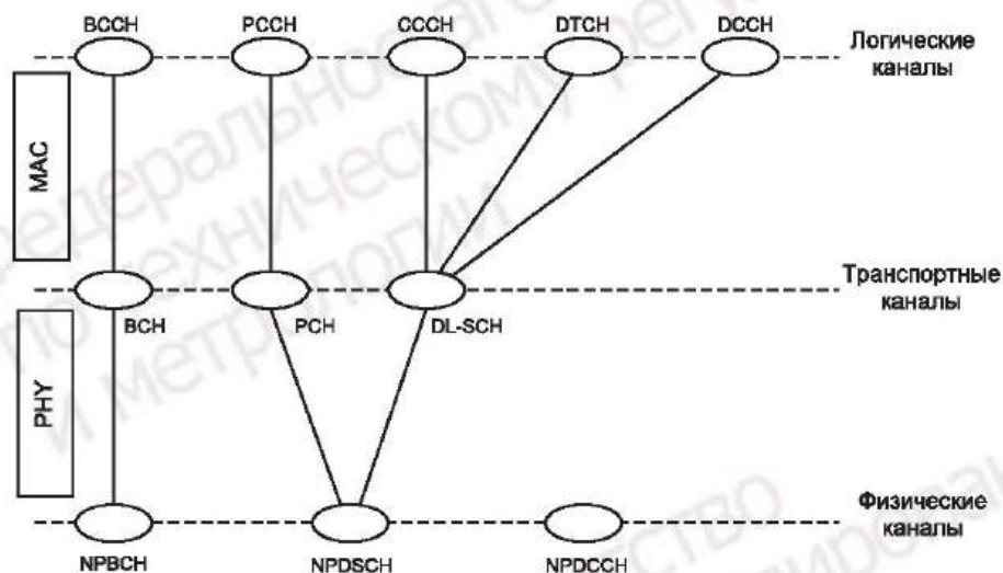
Рисунок 11 — Схема каналов в downlink-канале
