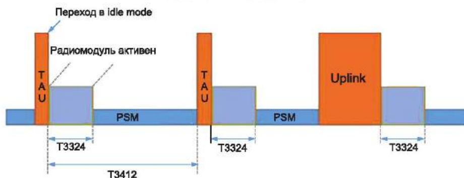
Рисунок 28 — Временная диаграмма режима энергосбережения PSM
