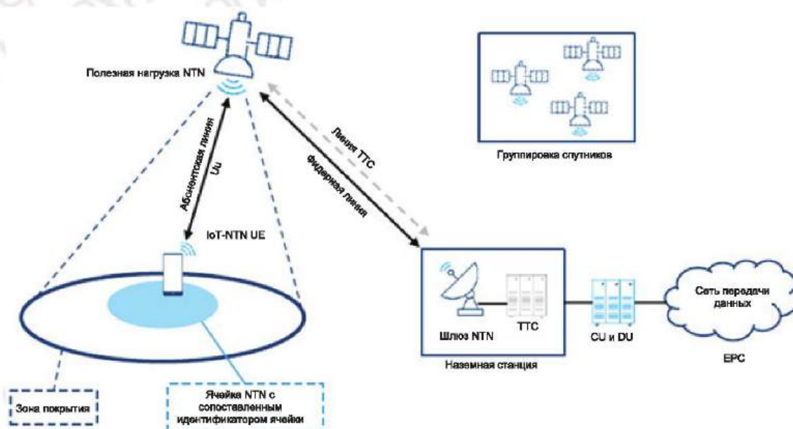
Рисунок 32 — Схема NTN-связи
