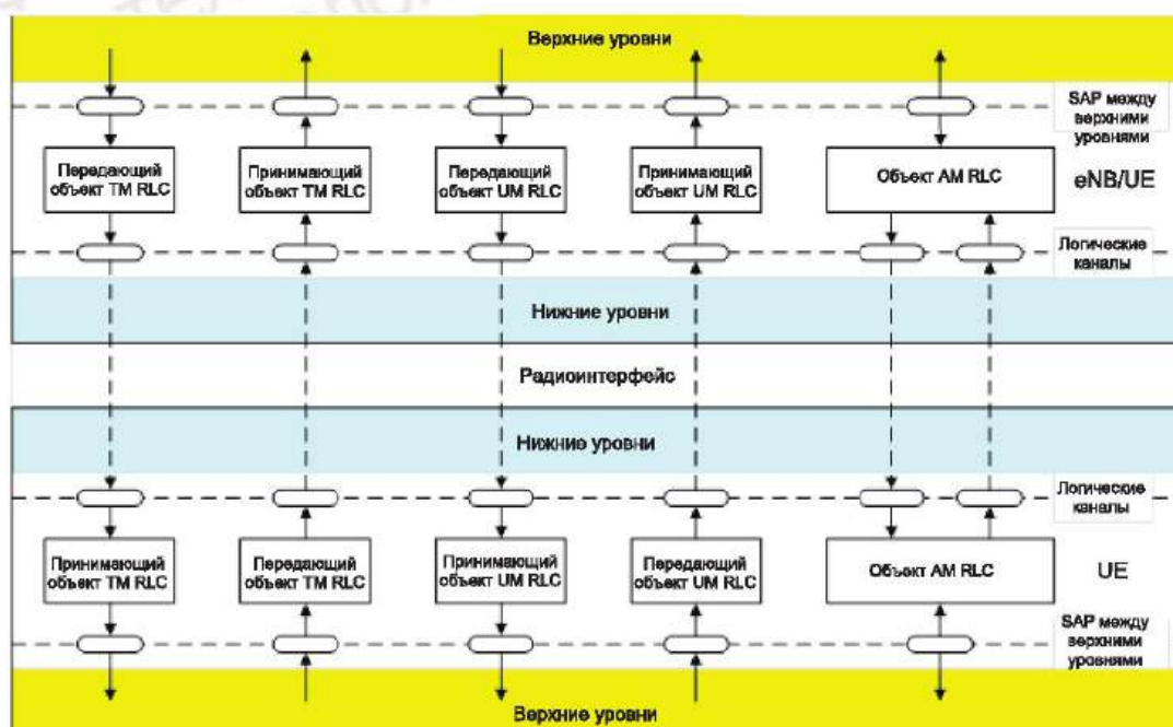
Рисунок 20 — Модель уровня RLC [9]
