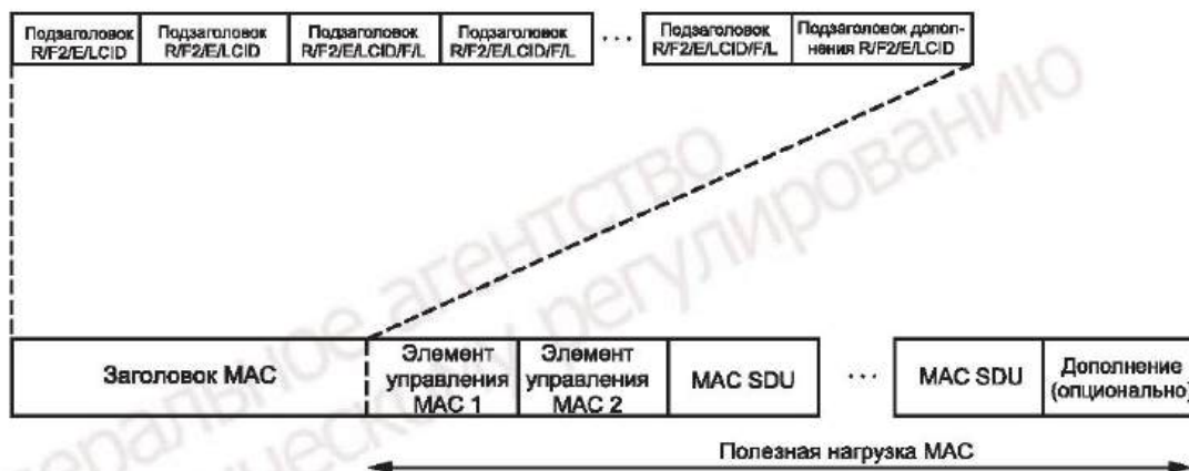
Рисунок 19 — Структура MAC PDU [8]
