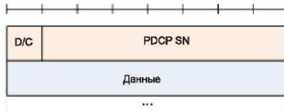
Рисунок 25 — PDCP PDU
