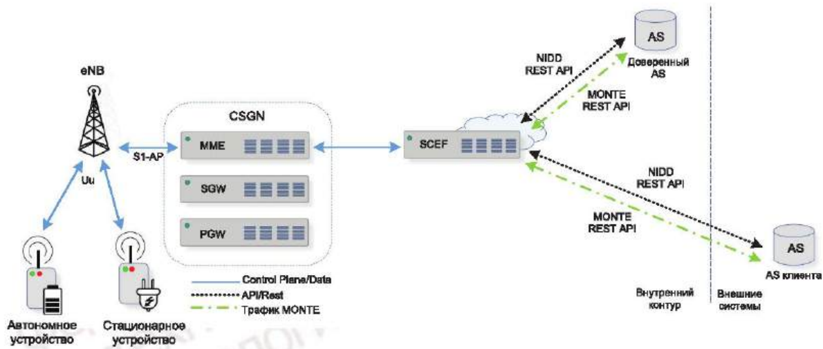
Рисунок 6 — Передача NIDD через SCEF
