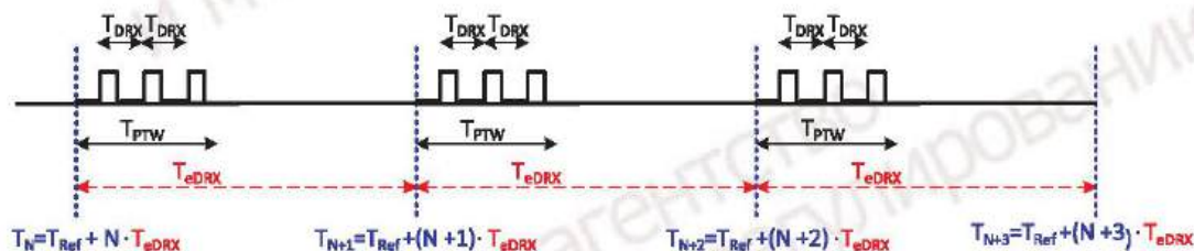
Рисунок 29 — Циклы расширенного режима прерывистого приема eDRX
