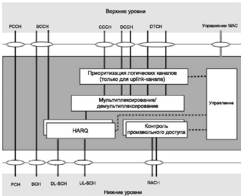
Рисунок 18 — Структура уровня MAC
