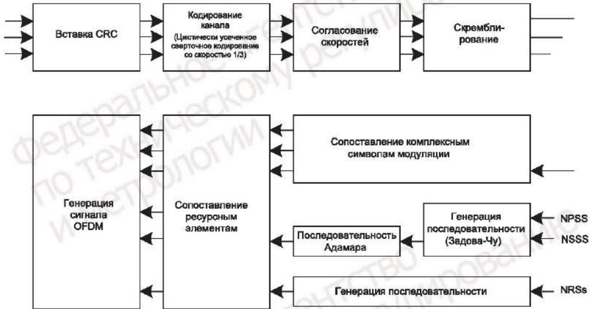
Рисунок 13 — Обработка физического downlink-канала
