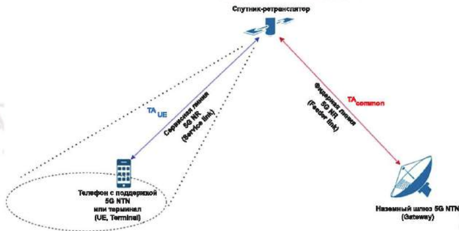
Рисунок 33 — Задержка распространения сигнала в NTN-сети
