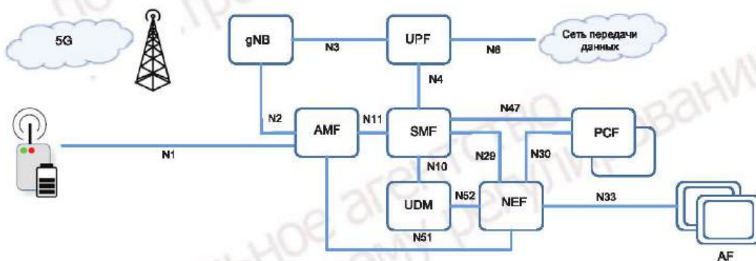
Рисунок 31 — Архитектура NB-IoT в сети 5G
