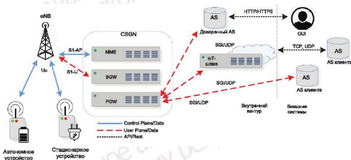
Рисунок 5 — Передача NIDD без SCEF через интерфейс SGi
