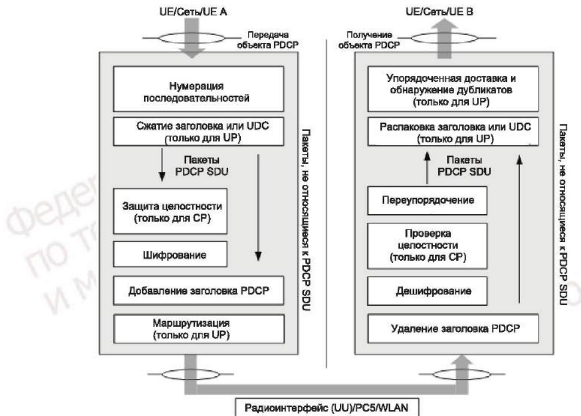
Рисунок 26 — Объект PDCP
