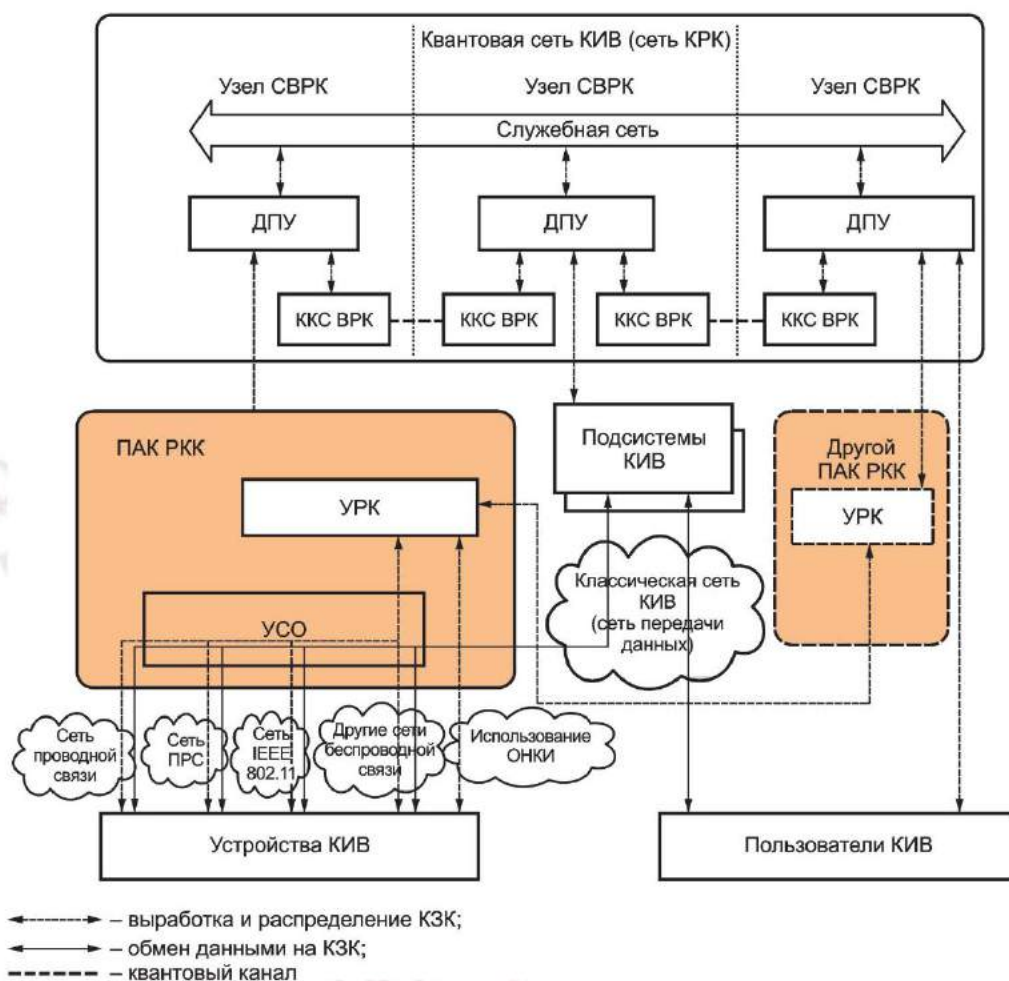
Рисунок 1 — Архитектура ПАК РКК и взаимодействующие с ПАК РКК элементы системы КИВ
