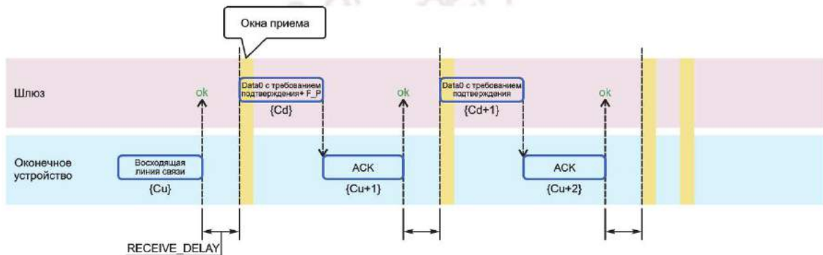
Рисунок 65 — Диаграмма передачи очереди нисходящих сообщений (пример 1)
