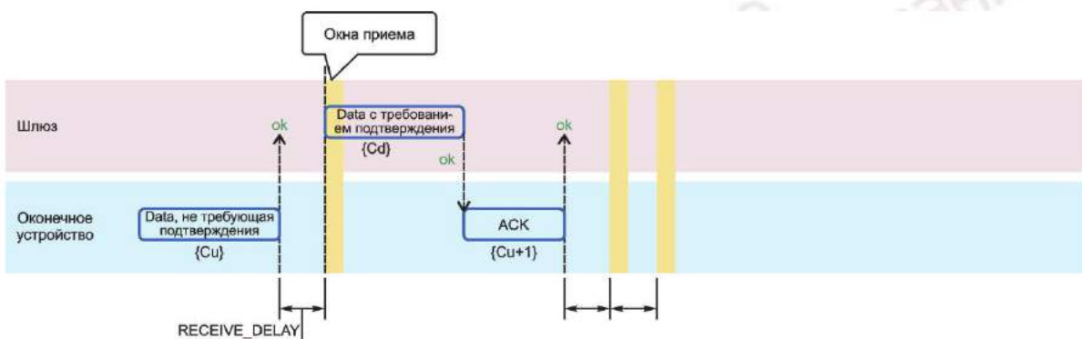
Рисунок 64 — Диаграмма передачи нисходящего сообщения с подтверждением
