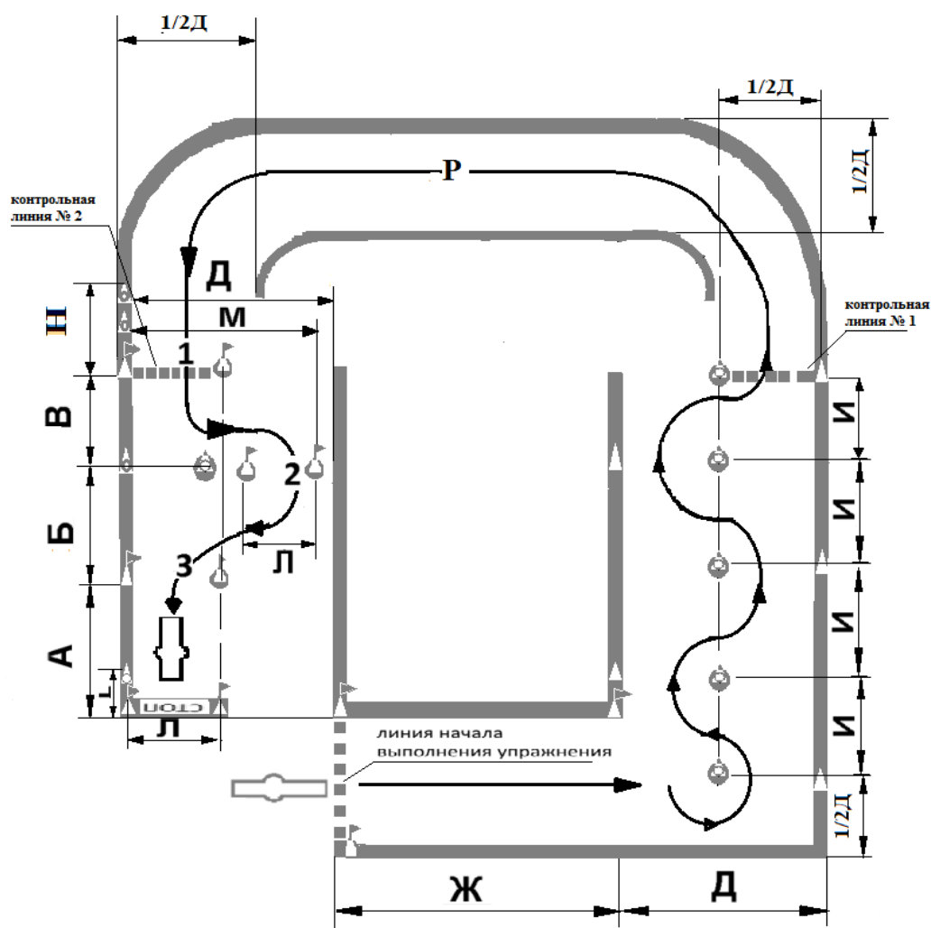
Схема «Б» элемента упражнения № 1 «Скоростное маневрирование».
